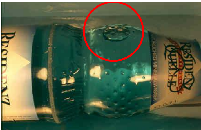
Abb. 3: Mandelkerngroße Dehnungsausgleichsluftblase
